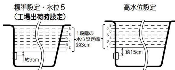
設定水位の目安
